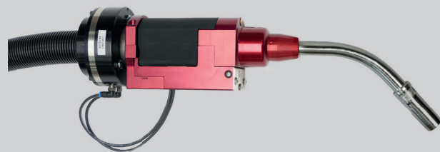
VWPR QE internt med MIG II 45 grader
