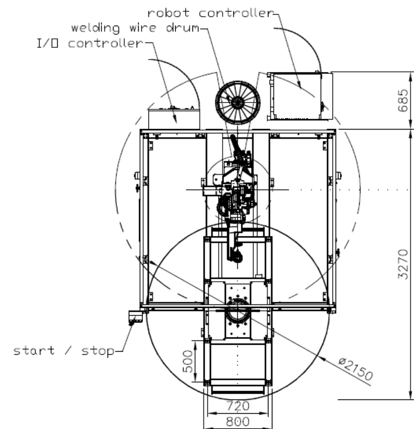
Dimensions de la cellule
