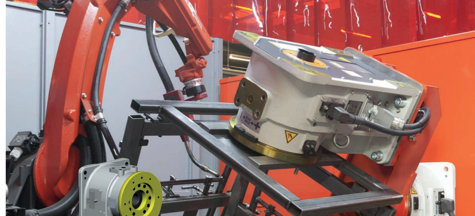
Pozycjoner POS250
