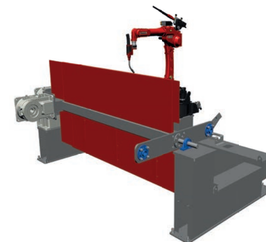
FRAME-C+FW (pariserhjul)
